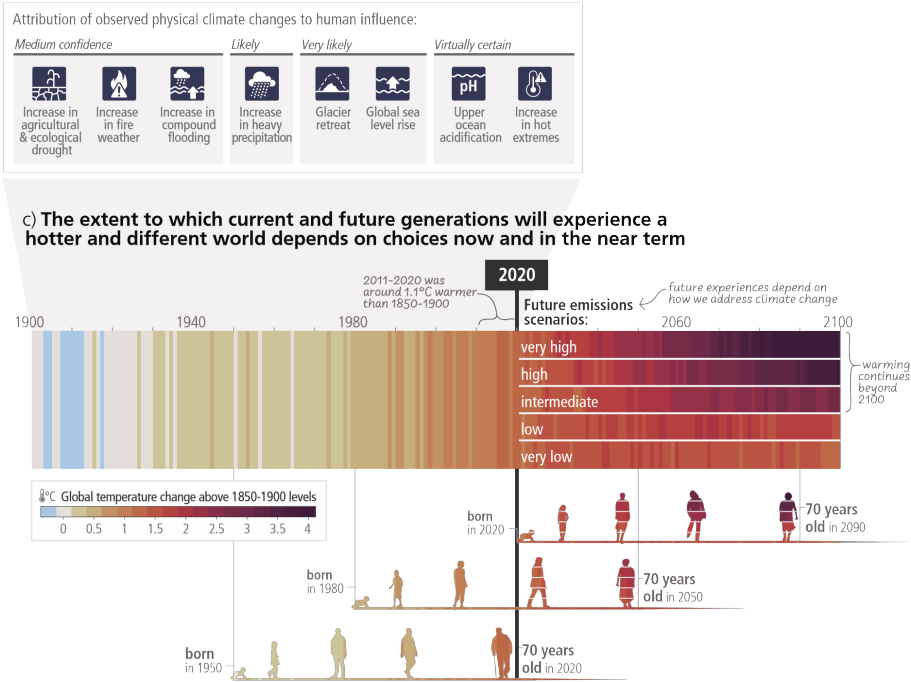
FIGURA 1. Evolución del calentamiento global
